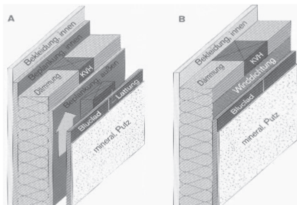
Schematische Darstellung bei der Verwendung von BLUCLAD als hinterlüftete Fassade ( A ) und als Direktbeplankung ( B )
