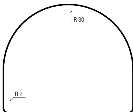
Profil-Nr. 117
