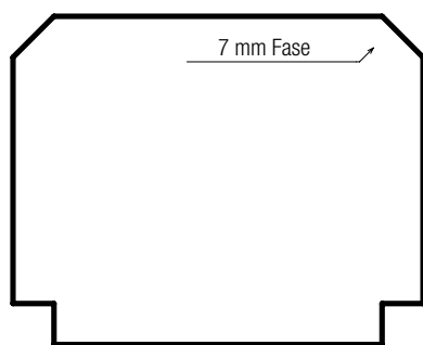
Profil-Nr. 88
