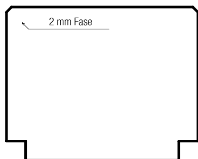
Profil-Nr. 78
