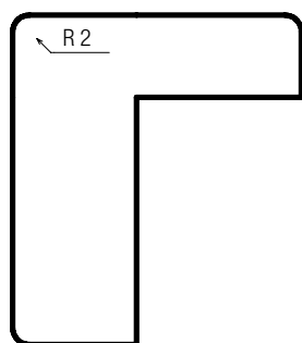
Profil-Nr. 108
