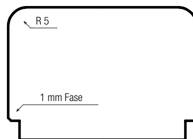
Profil-Nr. 115
