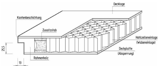
Innenleben einer Wabentür
