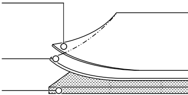
Melaminharzbeschichtung (Schutzfilm)
