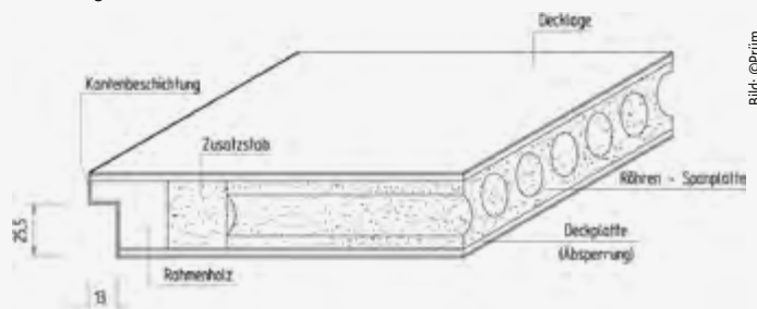
Innenleben einer Röhrenspantür
