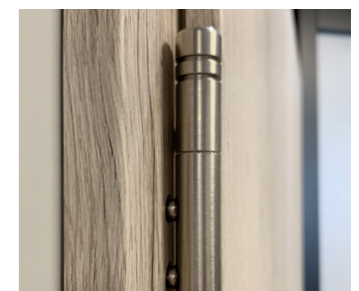
Ein 3-teiliges Band besteht aus drei Teilen. Der obere und untere Teil des Bandes mit jeweils nur einem Gewinde ist an die Tür verschraubt, das mittlere Teil mit zwei Schraub-Gewinden gehört an die Zarge. Verbunden werden diese Teile durch einen Stift.
