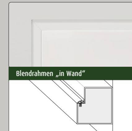
Puro 40 - Zarge in die Wand integriert
