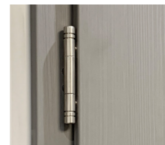
Ein 3-teiliges Band besteht aus drei Teilen. Der obere und untere Teil des Bandes mit jeweils nur einem Gewinde ist an die Tür verschraubt, das mittlere Teil mit zwei Schraub-Gewinden gehört an die Zarge. Verbunden werden diese Teile durch einen Stift.
