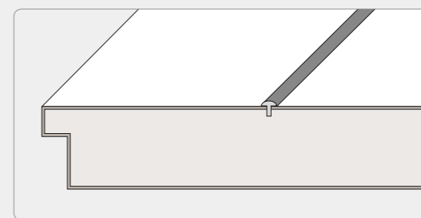
Der in verschiedenen Oberflächen erhältliche Linea-Keder wird in das Türblatt eingelegt.
