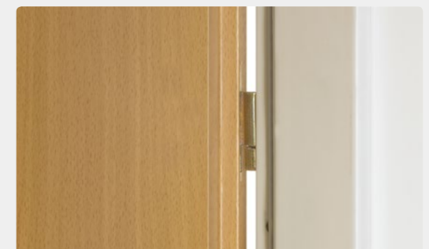
Detail TGL-Tür mit Fitschenband und Stahlzarge
