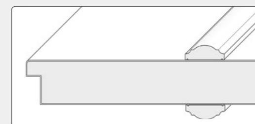
Türblatt mit aufgesetzten Leisten
